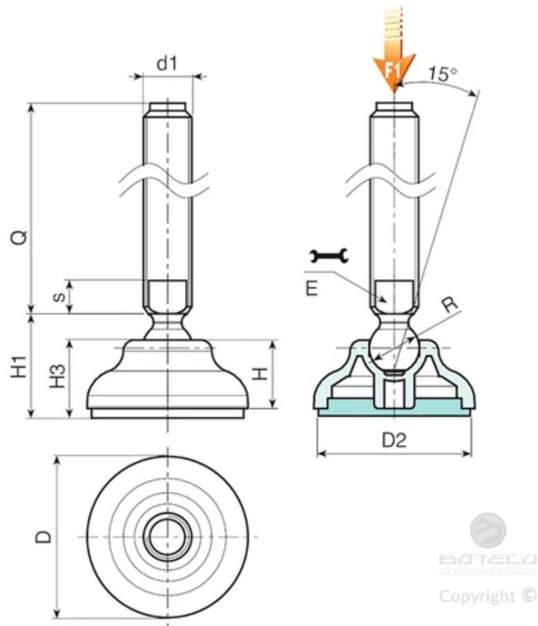
버전 P909: B형 스템(렌치용 밀링 시트 포함) 및 12,5 볼이 있는 장착 발 - SBS 미끄럼 방지 베이스 포함
