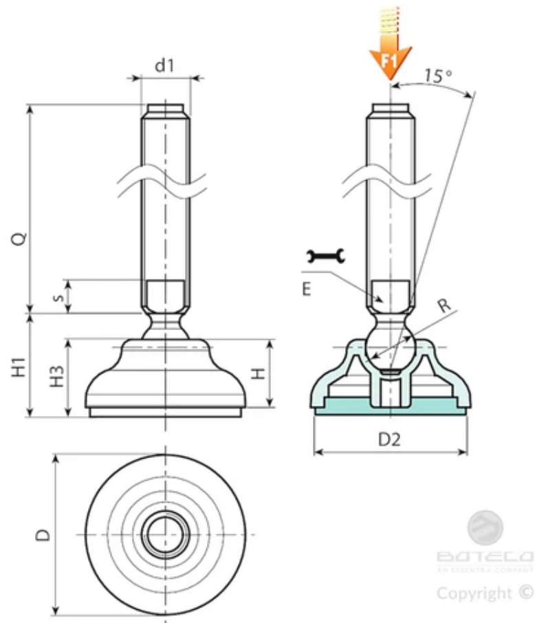
버전 P910: 스템 타입 B(렌치용 밀링 시트 포함) 및 볼 15가 있는 장착 발 - SBS 미끄럼 방지 베이스 포함
