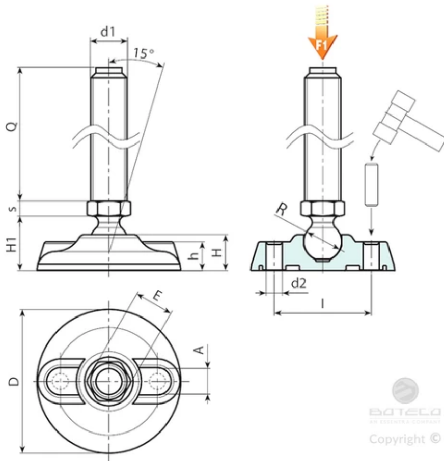
버전 P911: A형 스템(육각형 베이스 포함) 및 12,5 볼이 있는 장착 받침대
