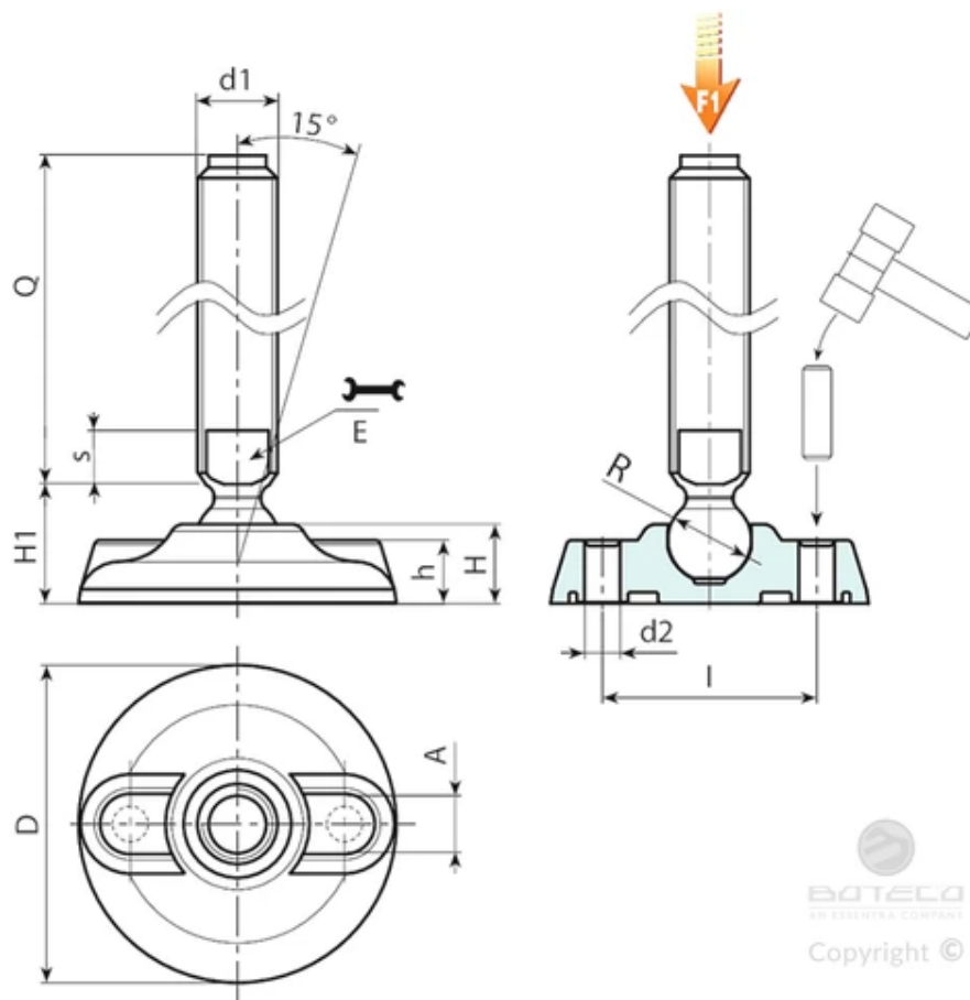
버전 P914: 스템 타입 B(렌치용 밀링 시트 포함) 및 볼 24가 있는 장착 발
