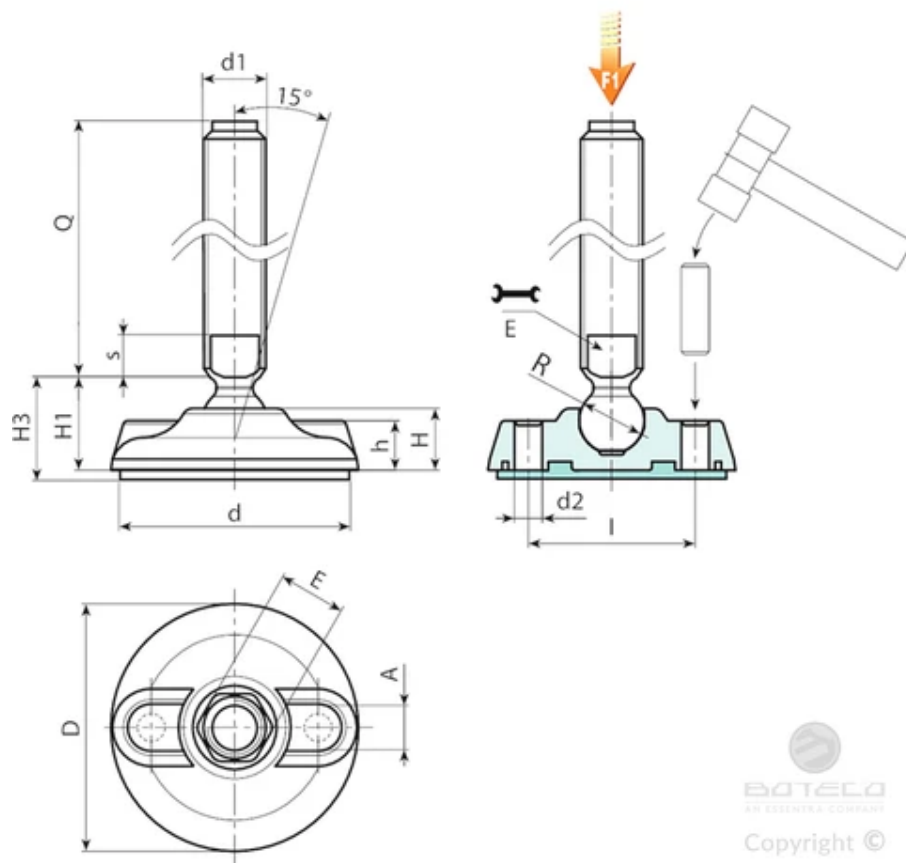
버전 P917: 스템 타입 B(렌치용 밀링 시트 포함) 및 볼 15가 있는 장착 발 - SBS 미끄럼 방지 베이스 포함
