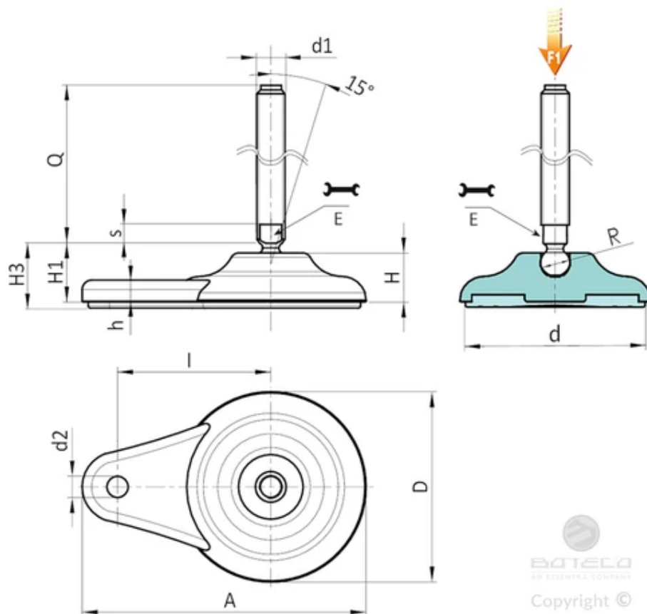
Ausführung P707: Gelenkfuß mit Verstellspindel Typ B - aus PA - (mit Aufnahme für Gabelschlüssel) und Kugel 15 - mit rutschfester Gummiauflage aus SBS
