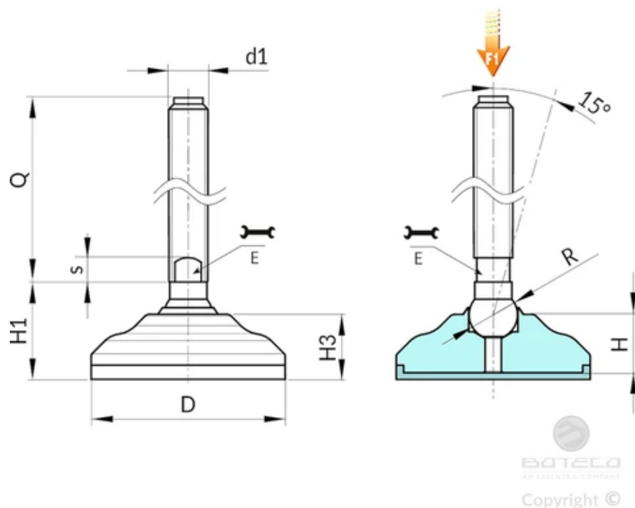
Ausführung P543: Gelenkfuß aus verzinktem Stahl mit Verstellspindel Typ B (mit Aufnahme für Gabelschlüssel) und Kugel 15 - mit rutschfester Gummiauflage aus TPV
