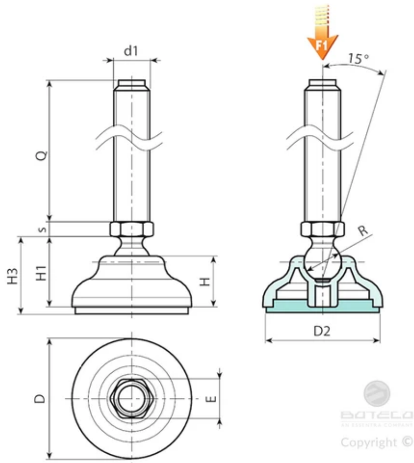
Ausführung P908: Gelenkfuß mit Verstellspindel Typ A (mit Aufnahme für Gabelschlüssel)-Kugel 15-mit rutschfester Gummiauflage aus SBS
