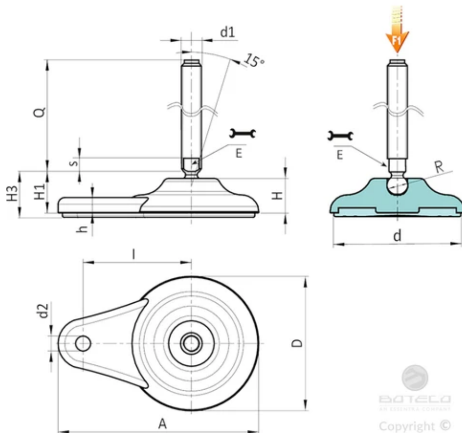
Ausführung P709: Gelenkfuß mit Verstellspindel Typ B - aus PA - (mit Aufnahme für Gabelschlüssel) und Kugel 24 - mit rutschfester Gummiauflage aus SBS
