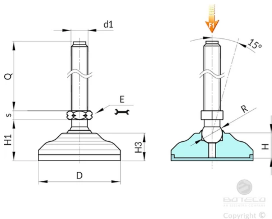
Ausführung P541: Gelenkfuß aus verzinktem Stahl mit Verstellspindel Typ A (mit Sechskant)-Kugel 15-mit rutschfester Gummiauflage aus TPV
