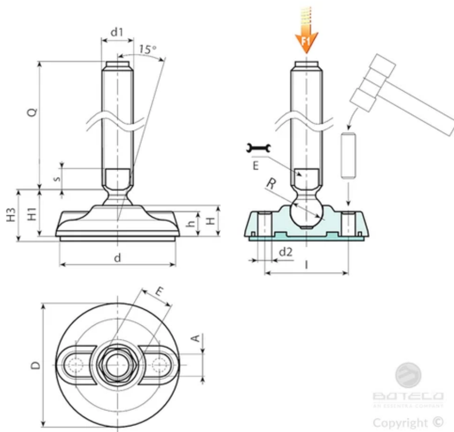
P918 változat: Rögzítőláb B típusú szárral (hornyolt foglalatnál a csavarkulcshoz) és 24 golyó - SBS csúszásmentes talppal
