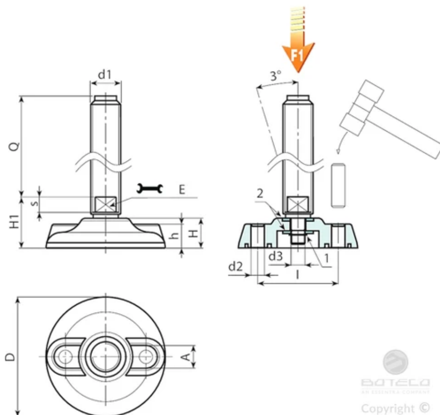
P801 változat: Rögzítőláb forgó szárral és rögzítőgyűrűvel rögzítve.
