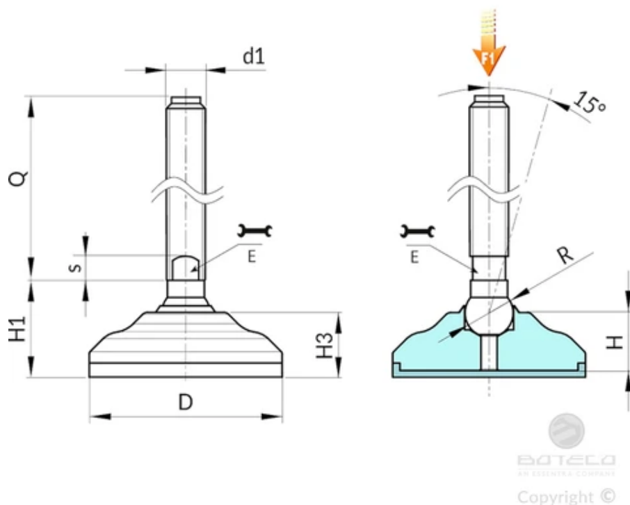
P543 változat: Horgonyzott acél rögzítőláb B típusú szárral (hornyolt foglalatnál a csavarkulcshoz) és 15 golyóval - TPV csúszásmentes talppal
