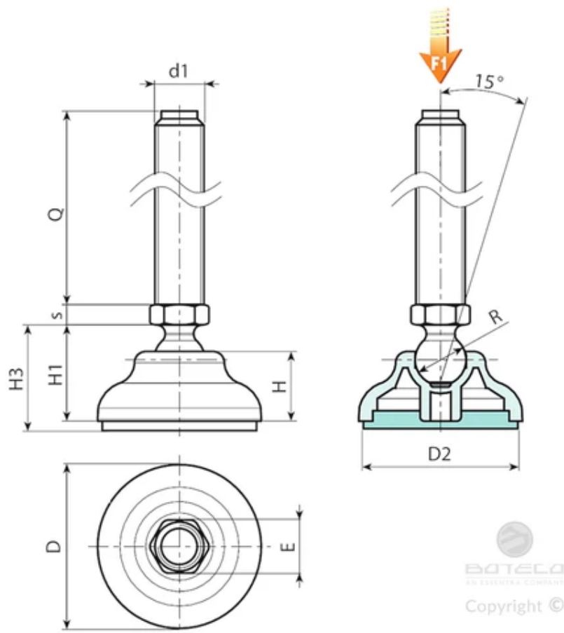
P908 változat: Rögzítőláb A típusú szárral (hatszögletű talppal) és 15 golyóval - SBS csúszásmentes talppal
