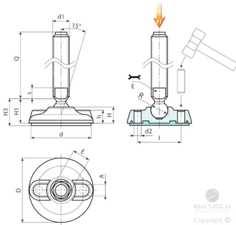
P917 változat: Rögzítőláb B típusú szárral (hornyolt foglalat a csavarkulcshoz) és 15 golyó - SBS csúszásmentes talppal
