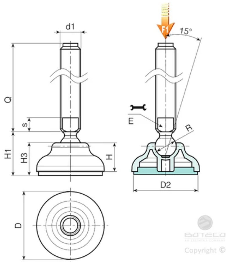
P909 változat: Rögzítőláb B típusú szárral (hornyolt foglalat a csavarkulcshoz) és 12,5 golyó - SBS csúszásmentes talppal
