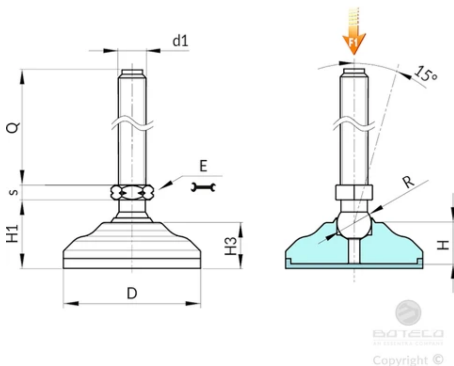
P541 változat: Horgonyzott acél rögzítőláb A típusú szárral (hatszögletű talppal) és 15 golyóval - TPV csúszásmentes talppal
