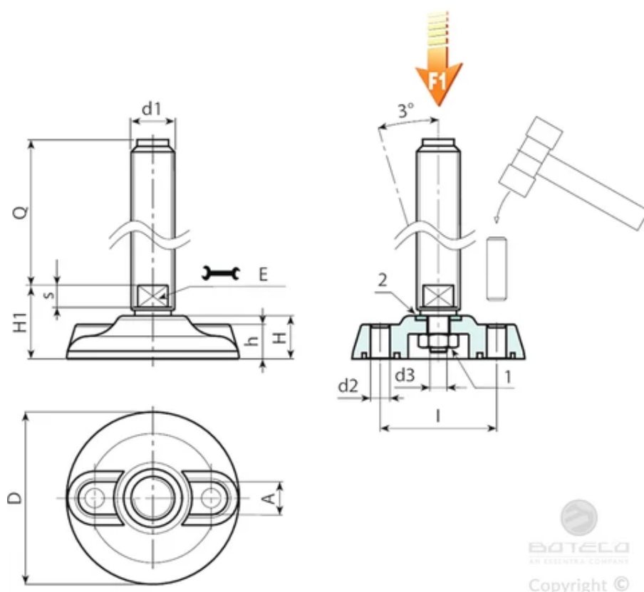
P800 változat: Rögzítőláb forgó szárral és anyával rögzítve.
