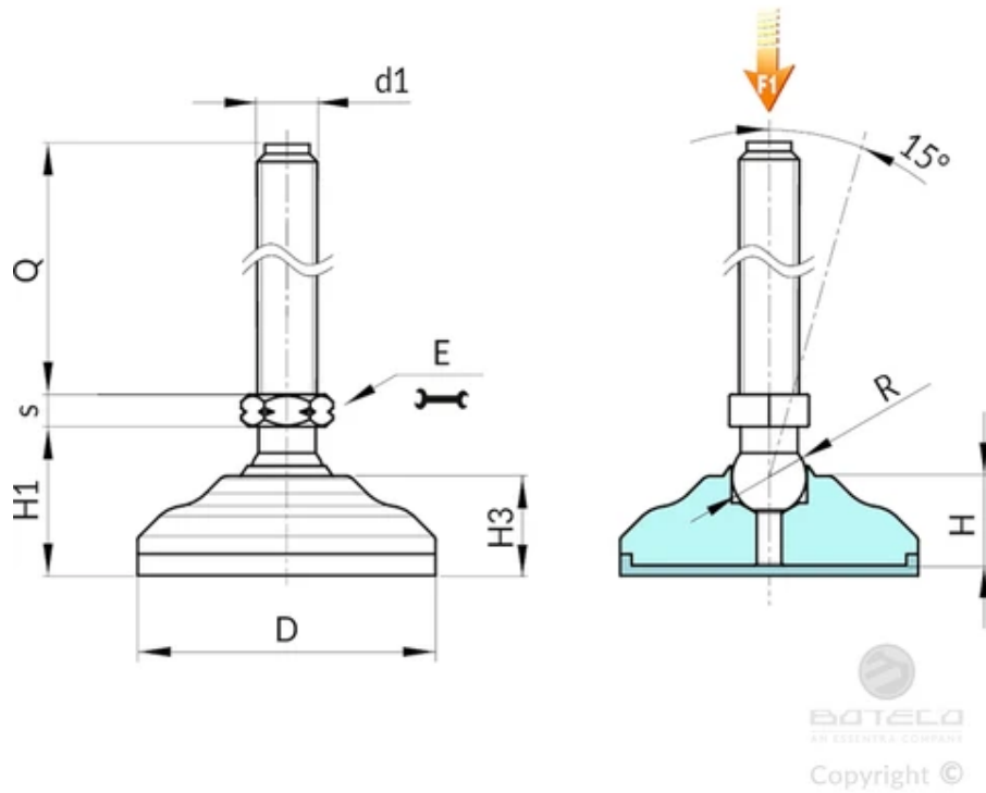
버전 P541: 아연 도금 스틸 장착 받침대(A형 스템, 육각형 베이스 및 15볼 포함) - TPV 미끄럼 방지 베이스 포함
