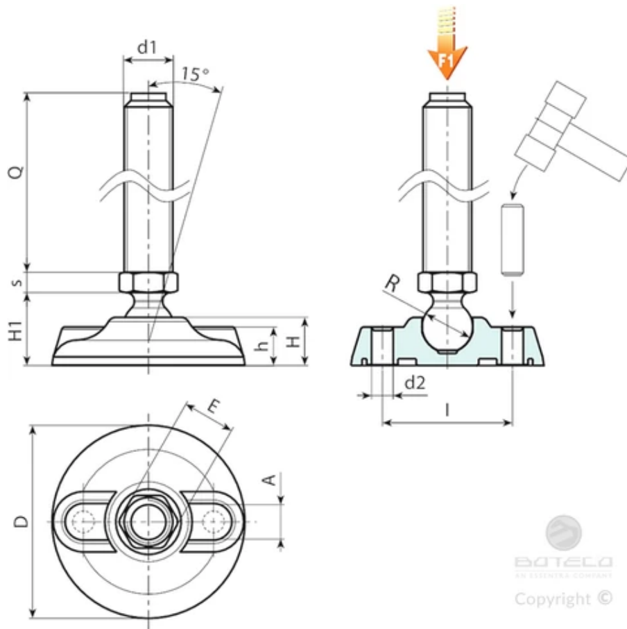
버전 P902: A형 스템(육각형 베이스 포함) 및 15볼이 있는 장착 받침대
