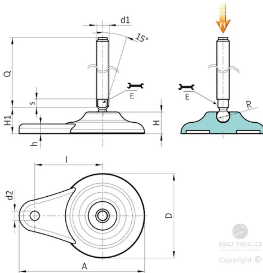
버전 P708: 지면 고정형 물방울 모양 장착 받침대 - 스템 타입 B (렌치용 밀링 시트 포함) 및 볼 24
