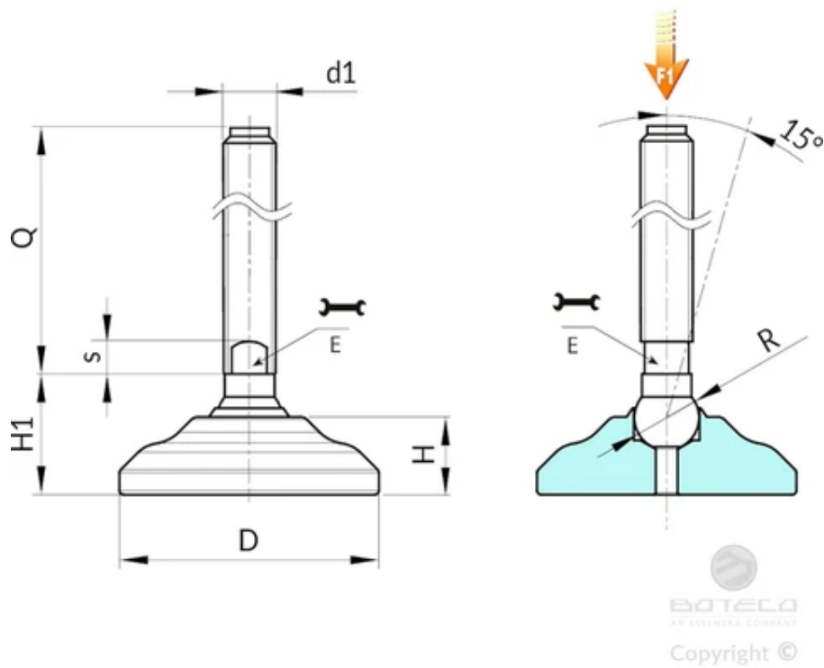
버전 P533: 아연 도금 스틸 장착 받침대, B형 스템(렌치용 밀링 시트 포함) 및 볼 15
