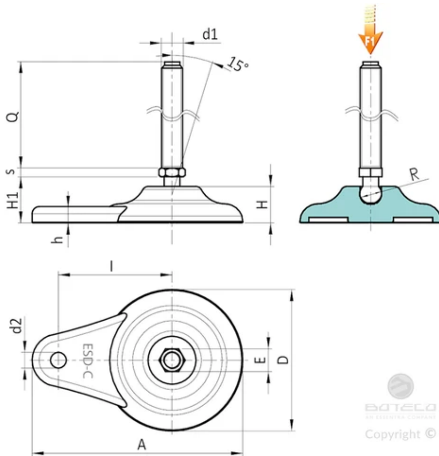
버전 P700ESD: A형 스템(육각형 베이스 포함) 및 12,5 볼이 있는 장착 받침대
