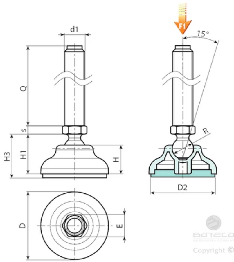
버전 P908: A형 스템(육각형 베이스 포함) 및 15볼이 있는 장착 받침대 - SBS 미끄럼 방지 베이스 포함
