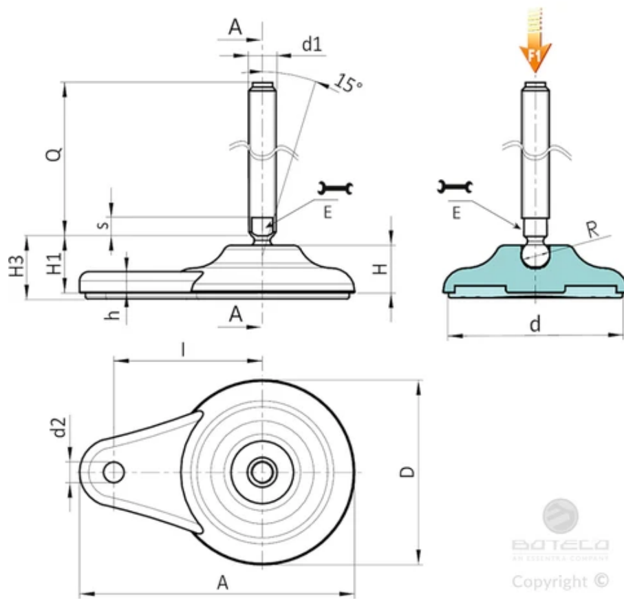
버전 P705: 물방울 모양 장착 받침대(지면 고정형) - 스템 타입 B(렌치용 홈 가공) 및 볼 12.5 - SBS 미끄럼 방지 베이스 포함
