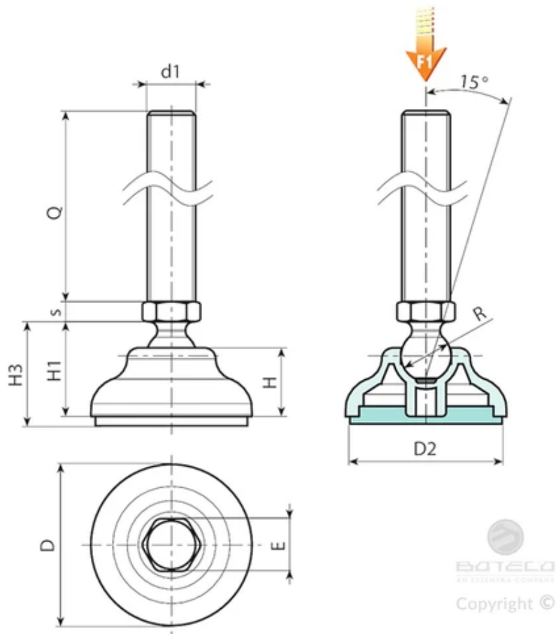
버전 P901: A형 스템(육각형 베이스 포함) 및 12,5 볼 베어링 장착 받침대 - SBS 미끄럼 방지 베이스 포함
