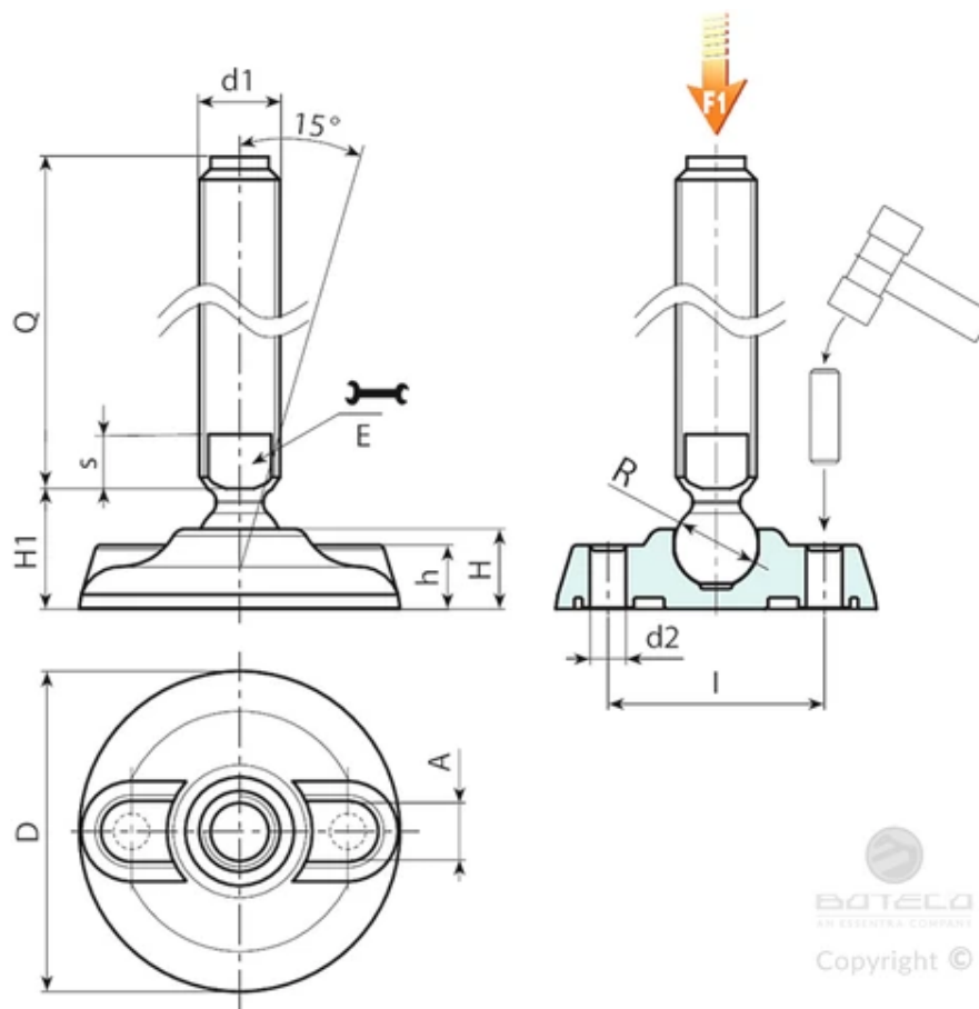
버전 P912: 스템 타입 B(렌치용 밀링 시트 포함) 및 볼 12,5 가 있는 장착 발
