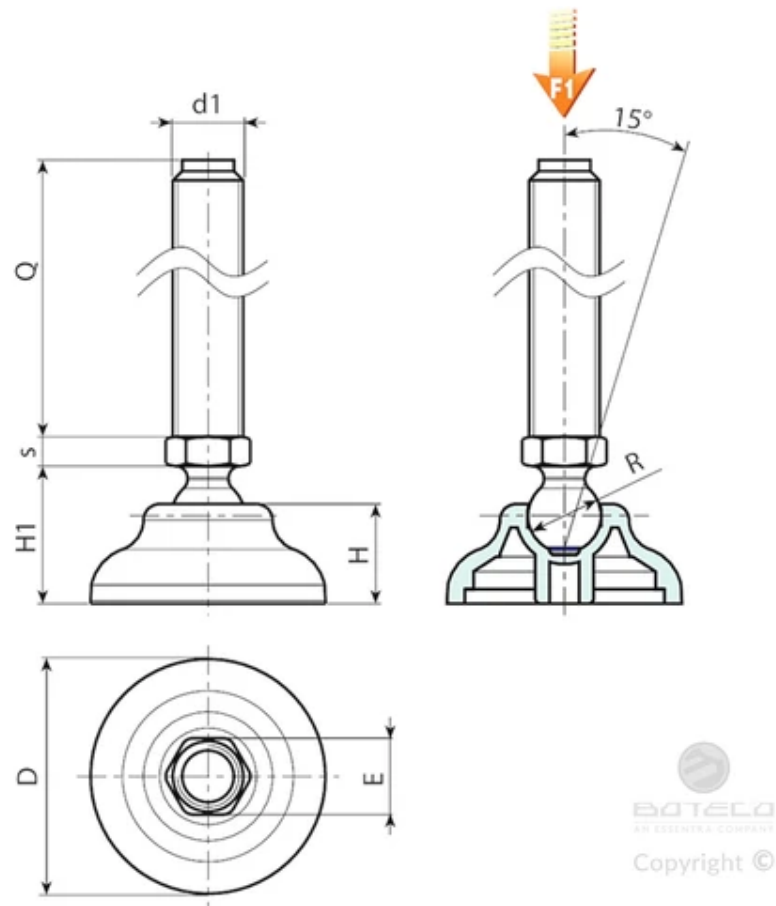
버전 P905: A형 스템(육각형 베이스 포함) 및 15볼이 있는 장착 받침대
