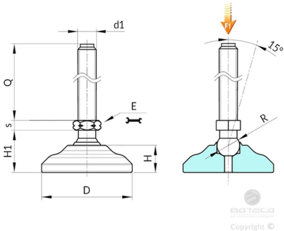
버전 P534: 아연 도금 스틸 장착 받침대, A형 스템(육각형 베이스 포함) 및 24볼
