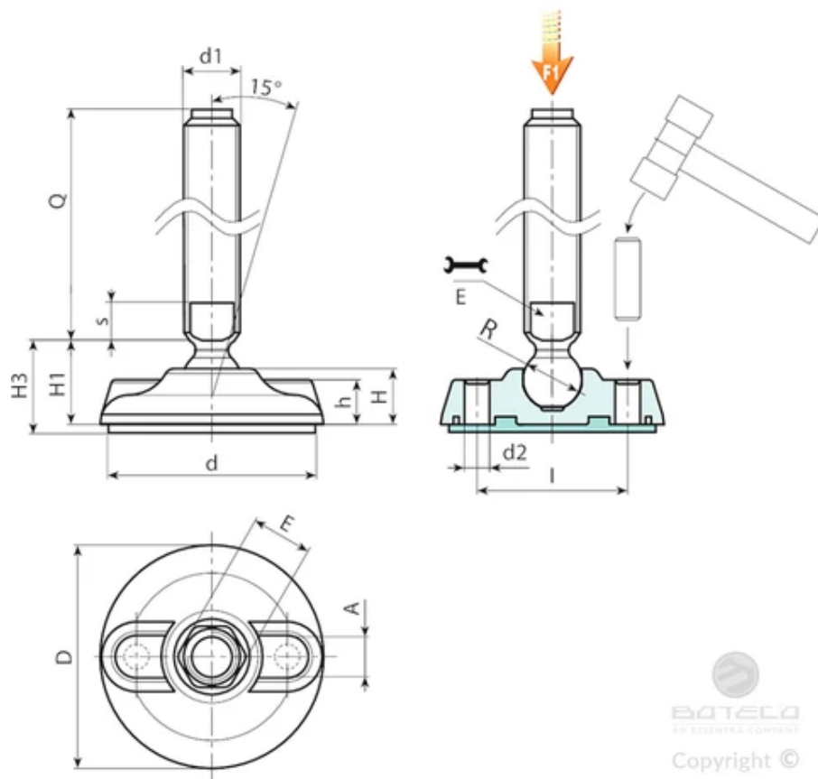
버전 P918: B형 스템(렌치용 밀링 시트 포함) 및 24볼이 있는 장착 발 - SBS 미끄럼 방지 베이스 포함
