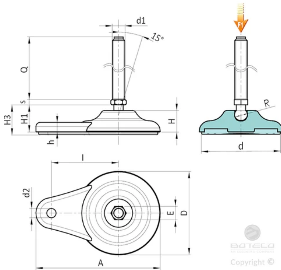
버전 P703: 물방울 모양 장착 받침대(지면 고정형) - 스템 타입 A(육각형 베이스 포함) 및 볼 15 - SBS 미끄럼 방지 베이스 포함
