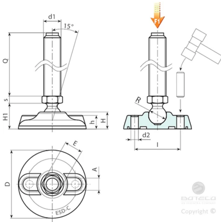
버전 P902ESD: A형 스템(육각형 베이스 포함) 및 15볼이 있는 장착 받침대
