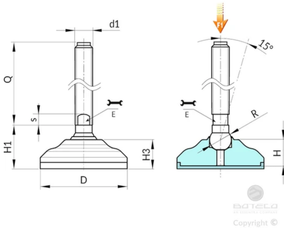
버전 P543: 아연 도금 스틸 장착 받침대(시스템 타입 B, 렌치용 밀링 시트 포함) 및 15볼 - TPV 미끄럼 방지 베이스 포함
