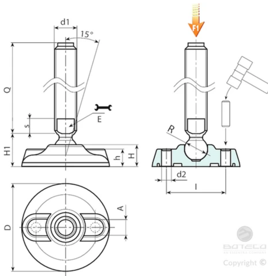
버전 P913: 스템 타입 B(렌치용 밀링 시트 포함) 및 볼 15가 있는 장착 발
