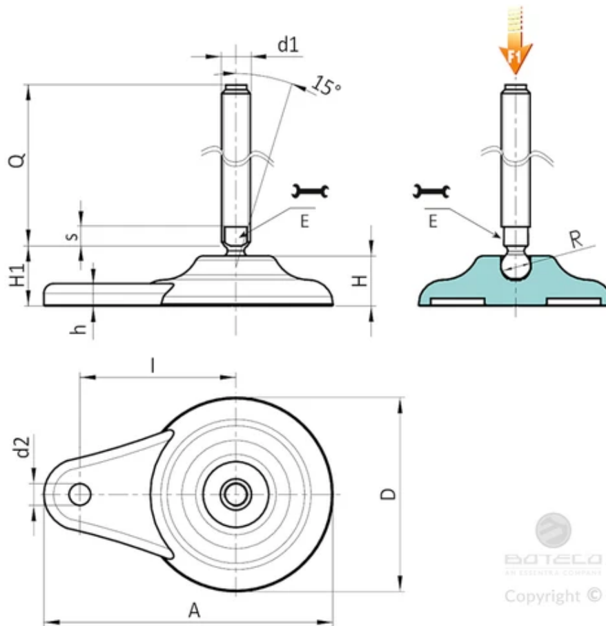
버전 P706: 지면 고정형 물방울 모양 장착 받침대 - 스템 타입 B (렌치용 밀링 시트 포함) 및 볼 15
