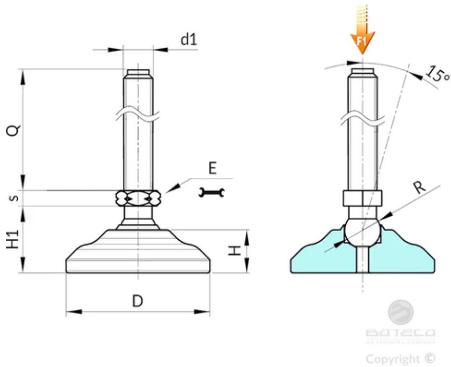
버전 P531: 아연 도금 스틸 장착 받침대, A형 스템(육각형 베이스 포함) 및 15볼
