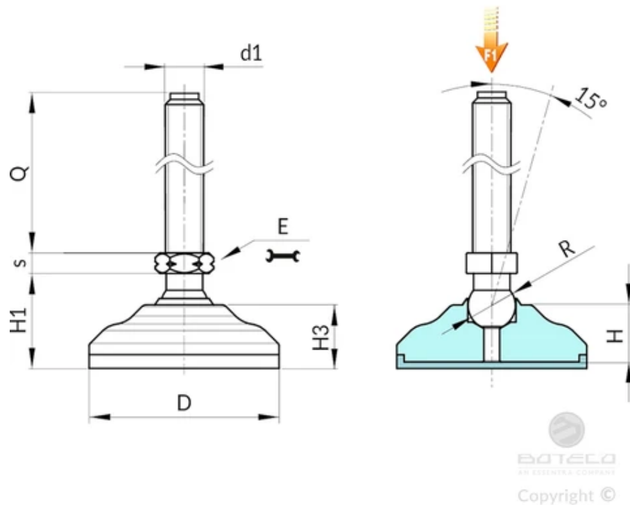
버전 P540: 아연 도금 스틸 장착 받침대, A형 스템(육각형 베이스 포함) 및 12,5 볼 - TPV 미끄럼 방지 베이스 포함
