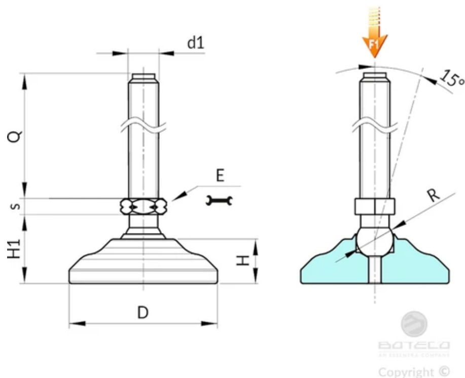
Versie P530: Stelvoet in verzinkt staal met draadeind type A (met zeskantbasis) en kogel 12,5.
