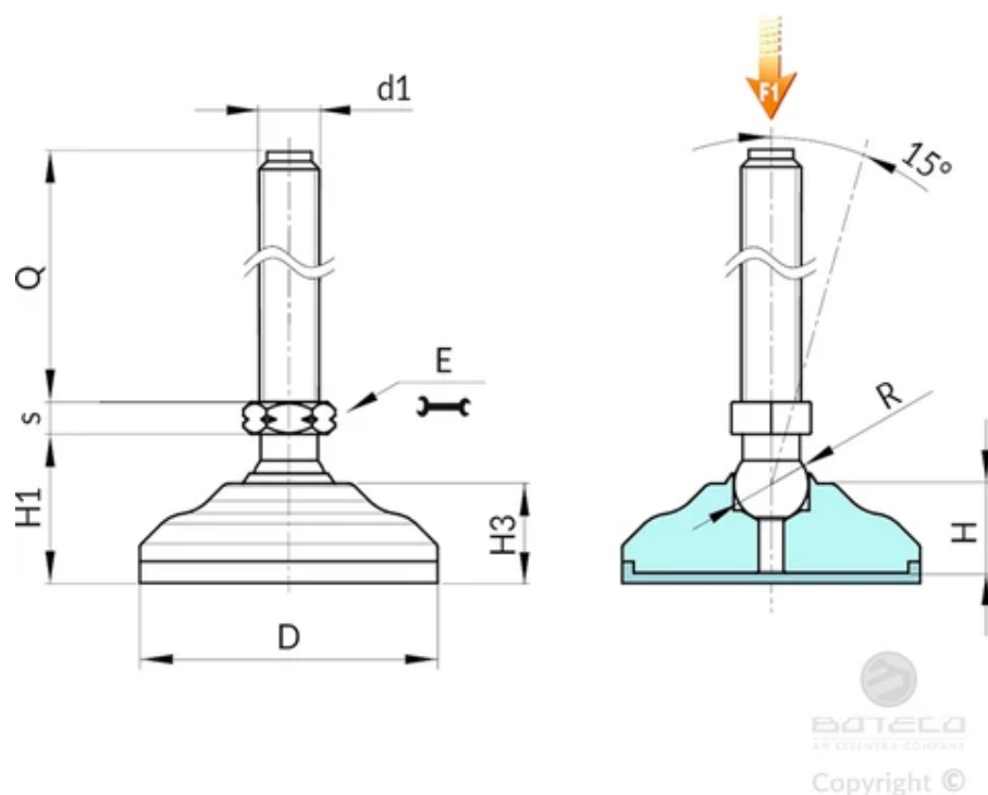
Versie P540: Stelvoet in verzinkt staal met draadeind type A (met zeskantbasis) en kogel 12,5 - antislipschijf in TPV.
