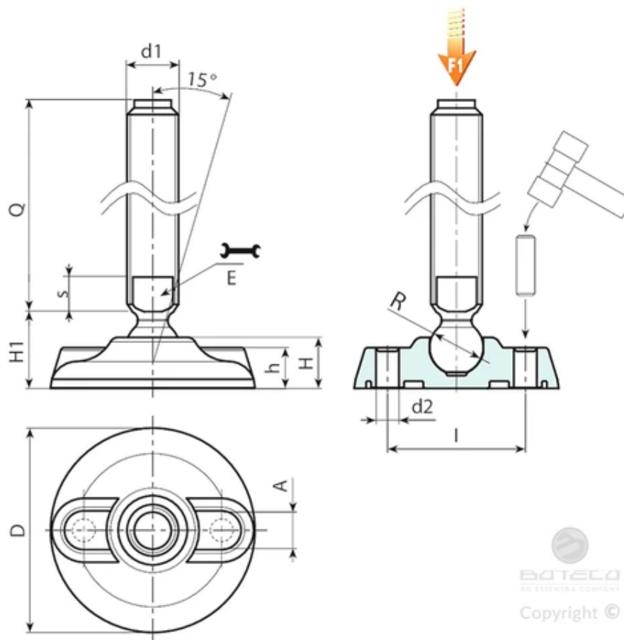
Versie P913: Stelvoet met draadeind type B (gefreesde zitting voor moersleutel) en kogel 15.
