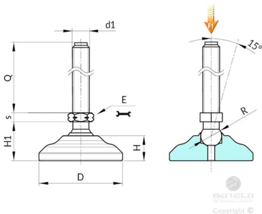
Версия P530: Опора из оцинкованной стали со стержнем типа А (с шестигранником) и шаровой головкой 12,5
