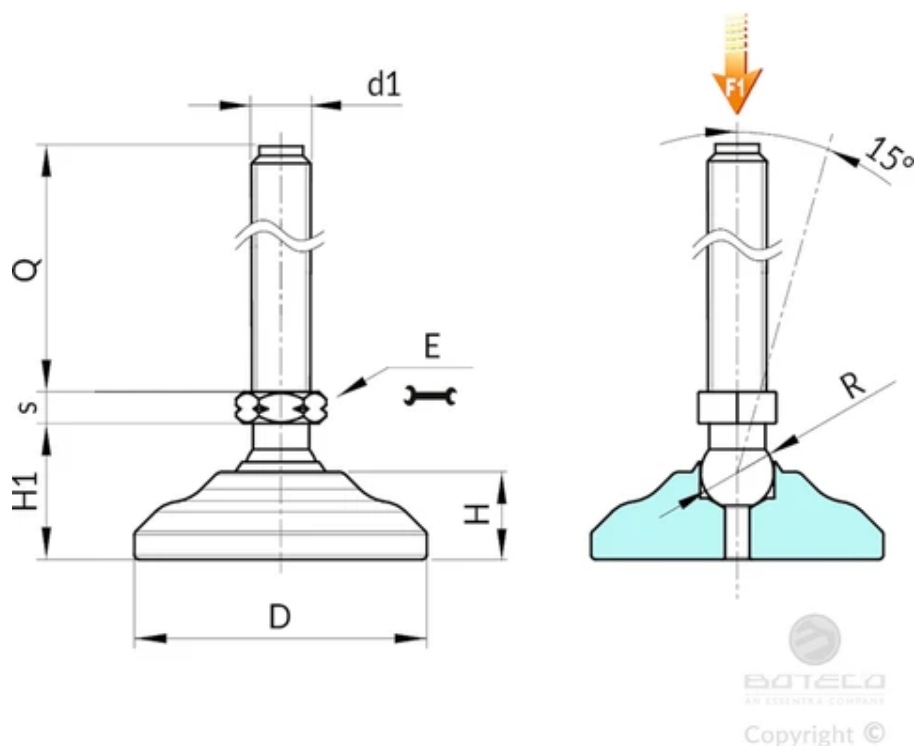
Версия P531: Опора из оцинкованной стали со стержнем типа А (с шестигранником) и шаровой головкой 15
