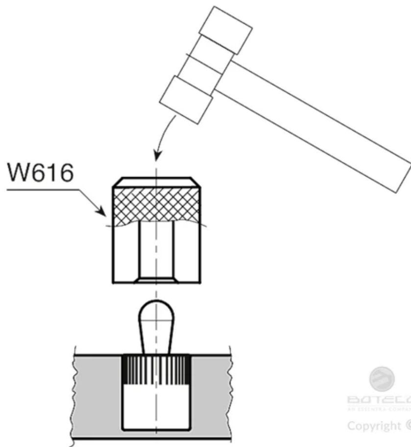
버전 W615: POM 노즐핀 및 싺이 있는 측면 스프링 플런저
